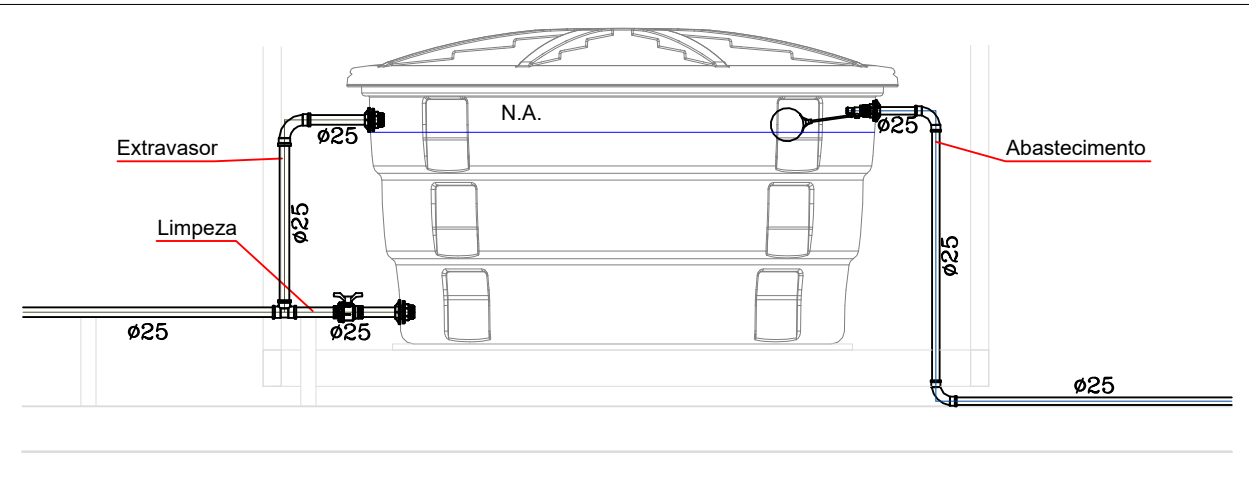
DETALHES GENÉRICO CAIXA D'AGUA - EXTRAVASOR, LIMPEZA E ABASTECIMENTO SEM ESCALA
