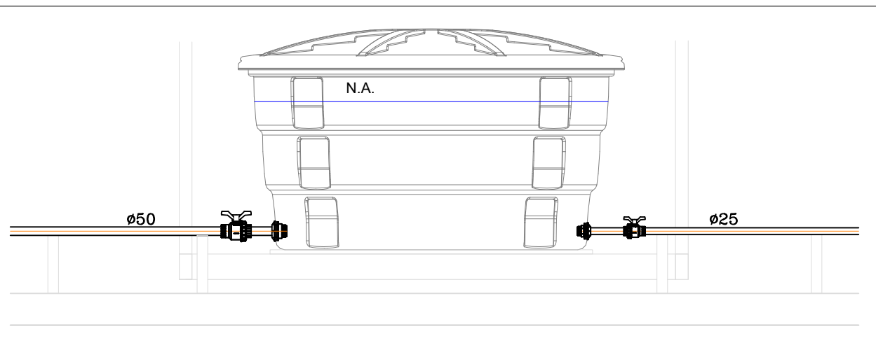
DETALHES GENÉRICO CAIXA D'AGUA - DISTRIBUIÇÃO SEM ESCALA
