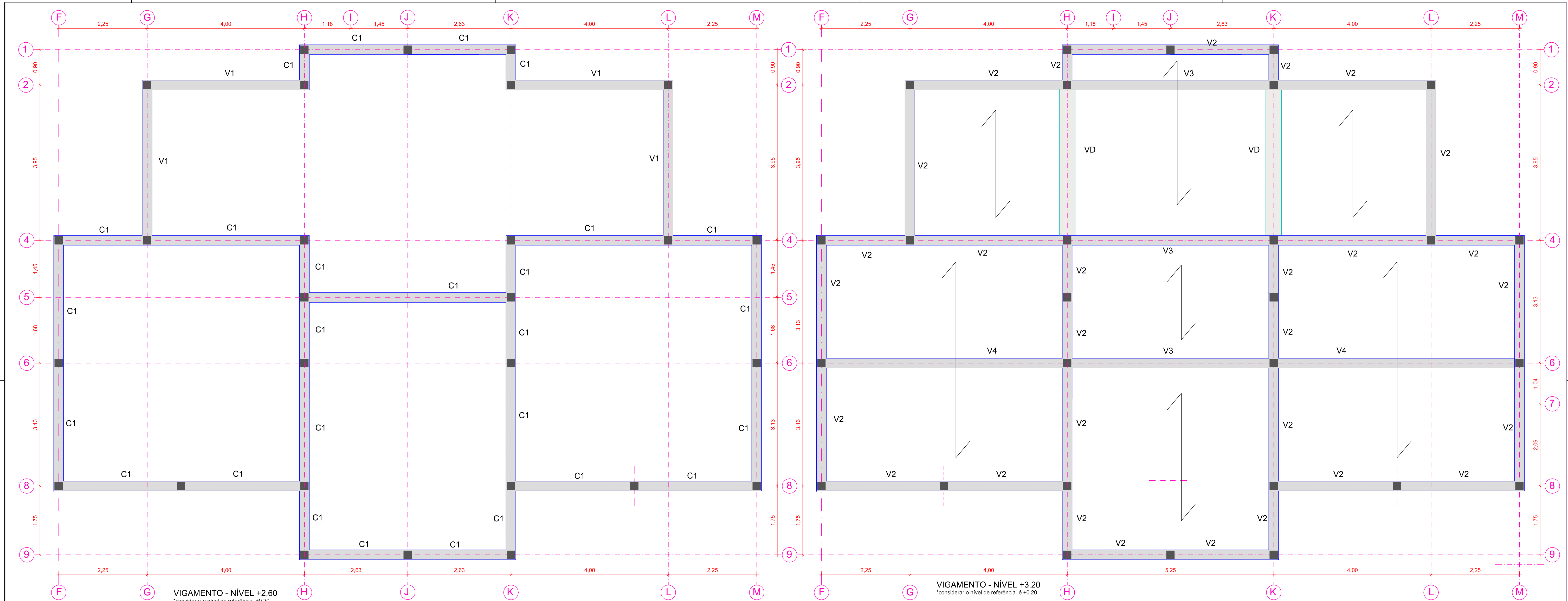
VIGAMENTO - NÍVEL +2.60 *considerar o nível de referência +0.20
