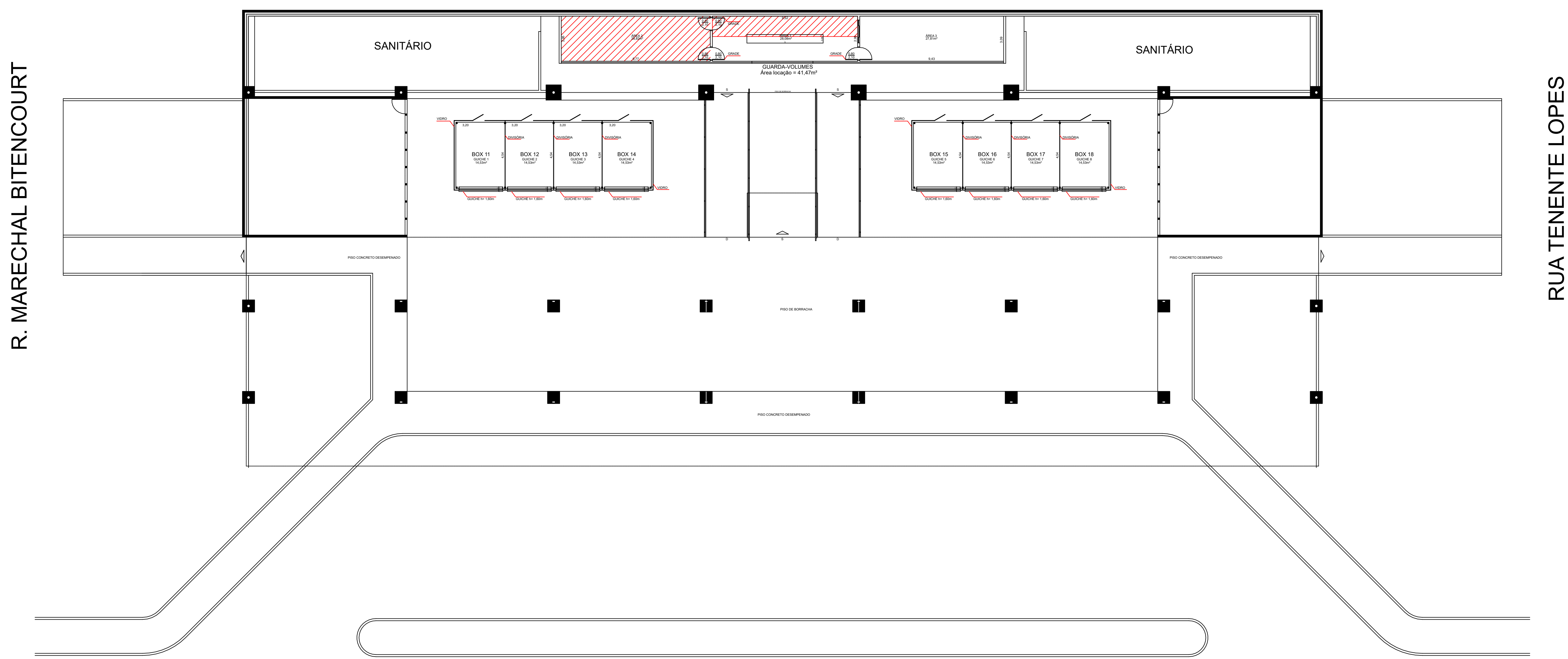
PLANTA - TERREO ESC.: 1/150
