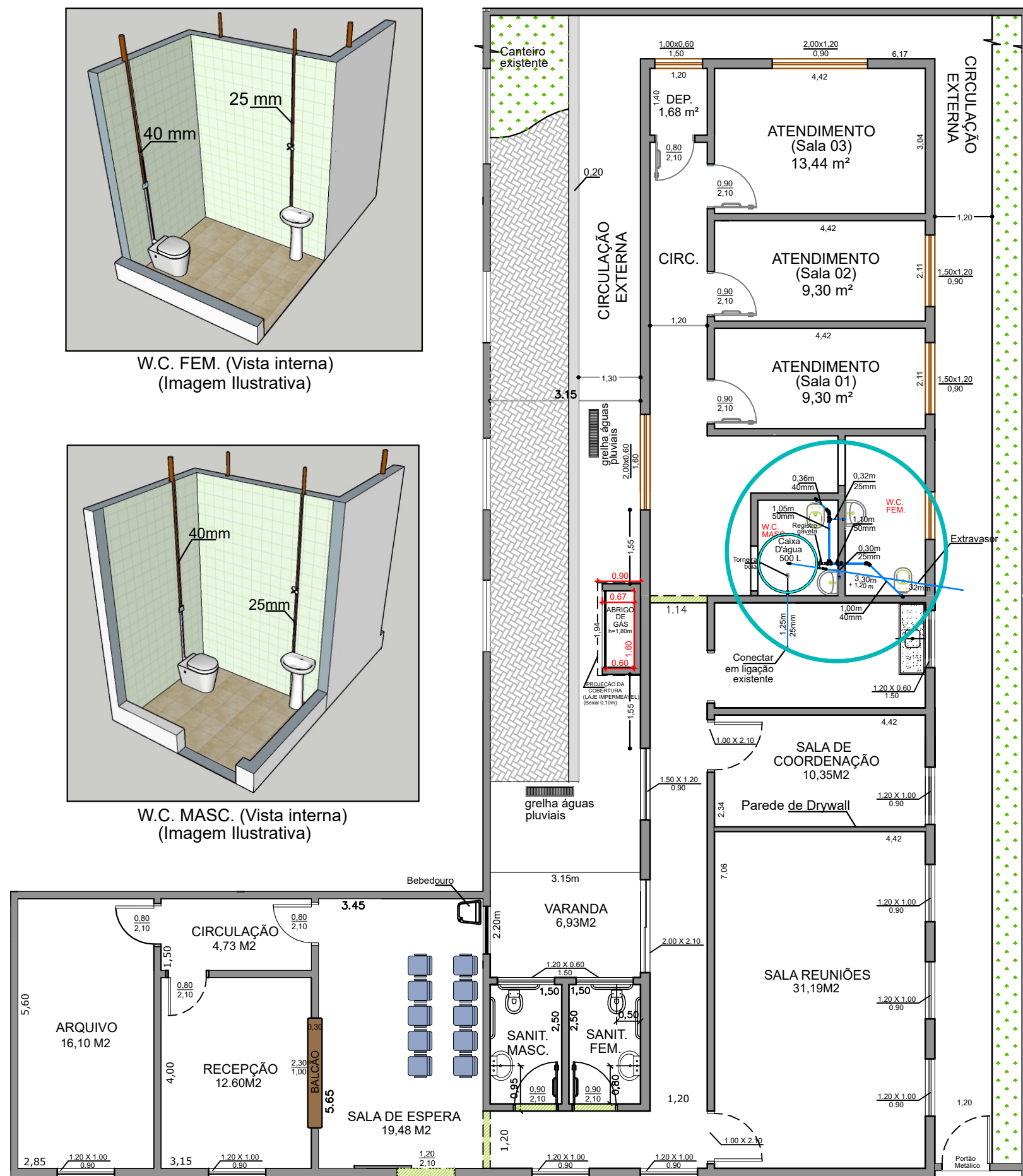
PLANTA BAIXA: (Pós reforma) Escala 1:100
