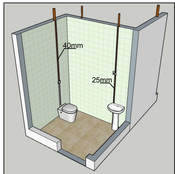
W.C. MASC. (Vista interna) (Imagem Ilustrativa)
