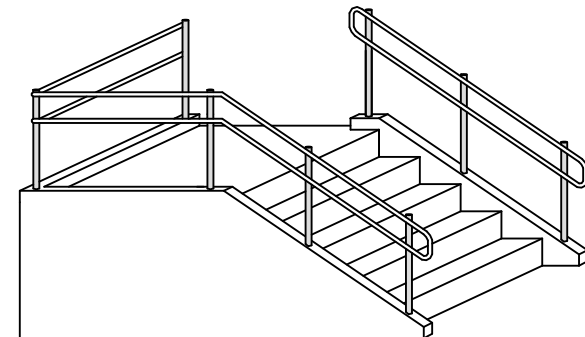
DETALHE 01 - ESCADA E CORRIMÃO Escala 1:50
