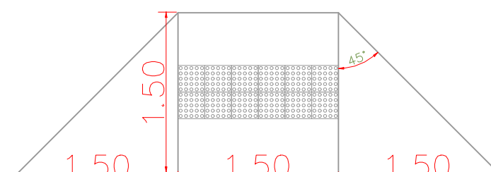
DETALHE 02 - RAMPA DE ACESSO Escala 1:50
