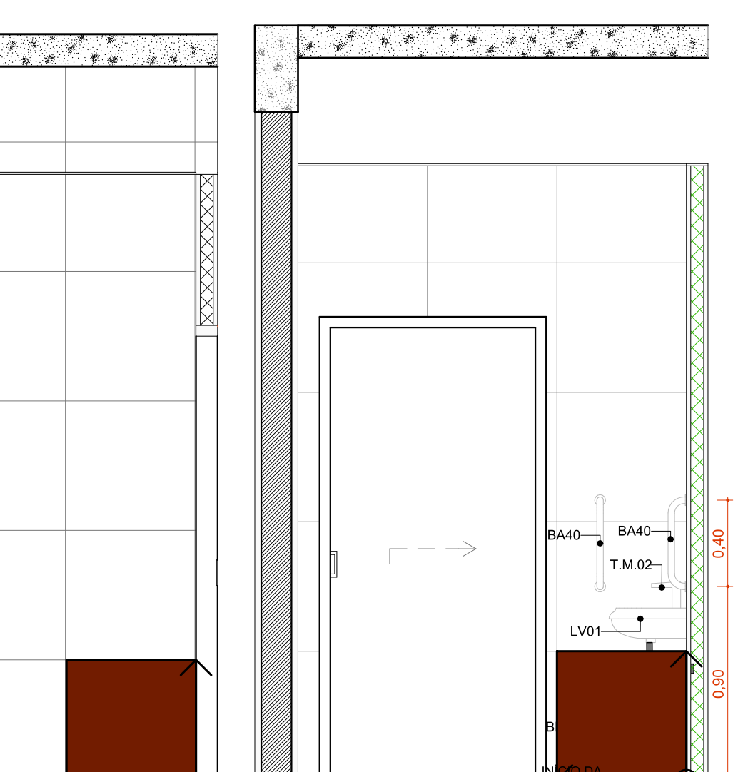
A.M.10 VISTA 3 Escala:1:25
