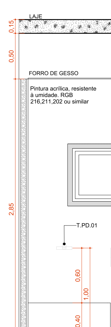
A.M.12 VISTA 2 Escala:1:25
