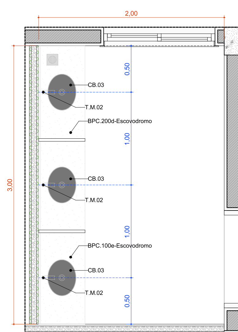
A.M.13 Escovodromo Escala:1:25
