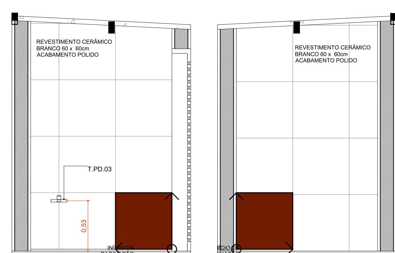
A.M.14 VISTA 3 Escala:1:25
