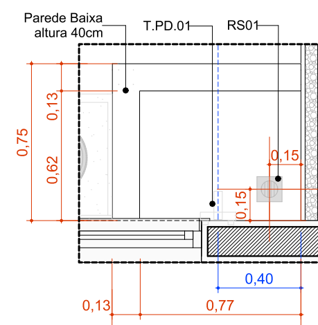
A.M.12 Higienização dos pés Escala:1:25
