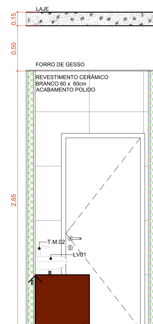
A.M.09 VISTA 2 Escala:1:25
