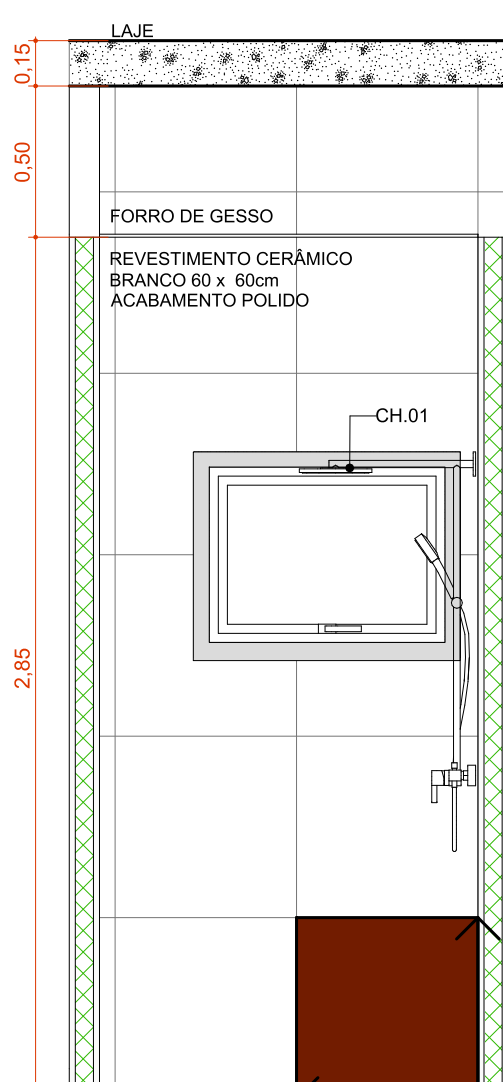
A.M.09 VISTA 1 Escala:1:25
