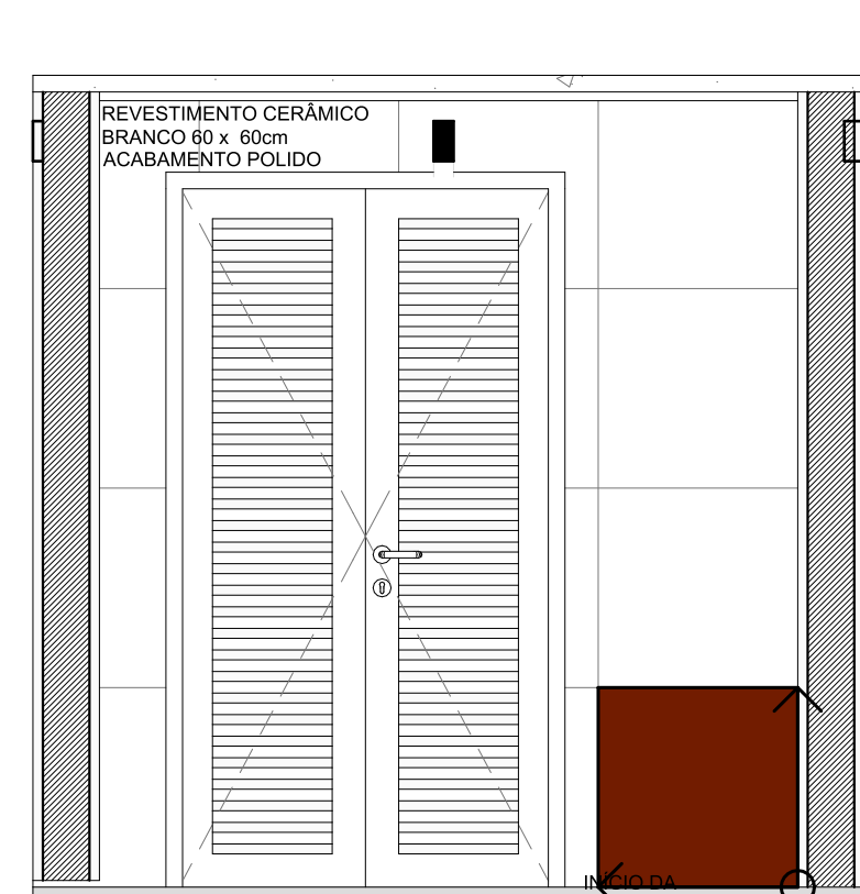
A.M.14 VISTA 1 Escala:1:25
