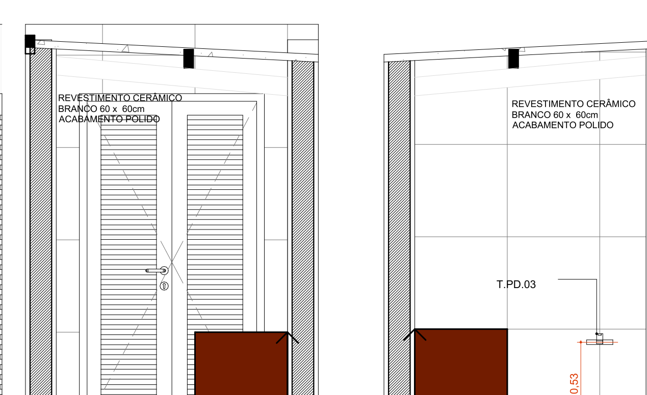
A.M.15 VISTA 3 Escala:1:25
