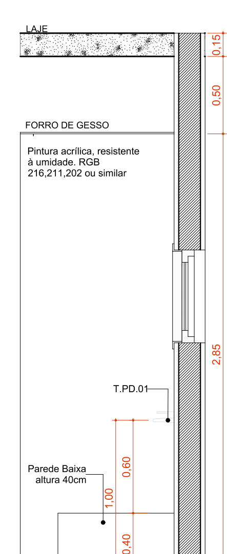
A.M.12 VISTA 1 Escala:1:25
