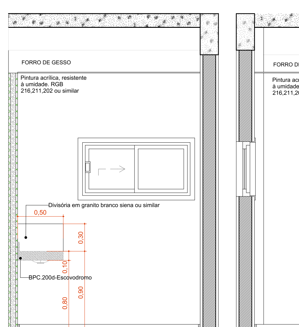
A.M.13 VISTA 1 Escala:1:25
