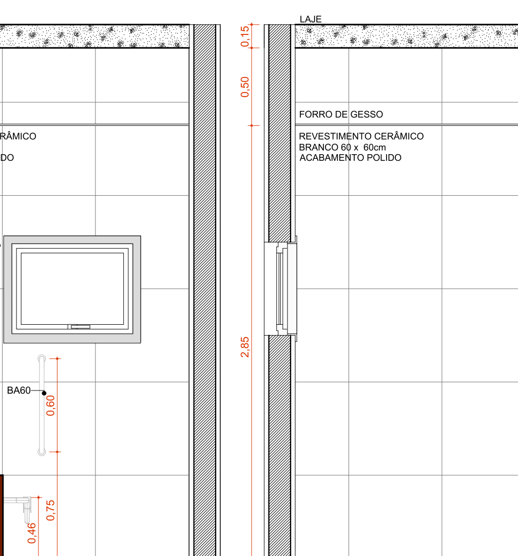
A.M.10 VISTA 2 Escala:1:25
