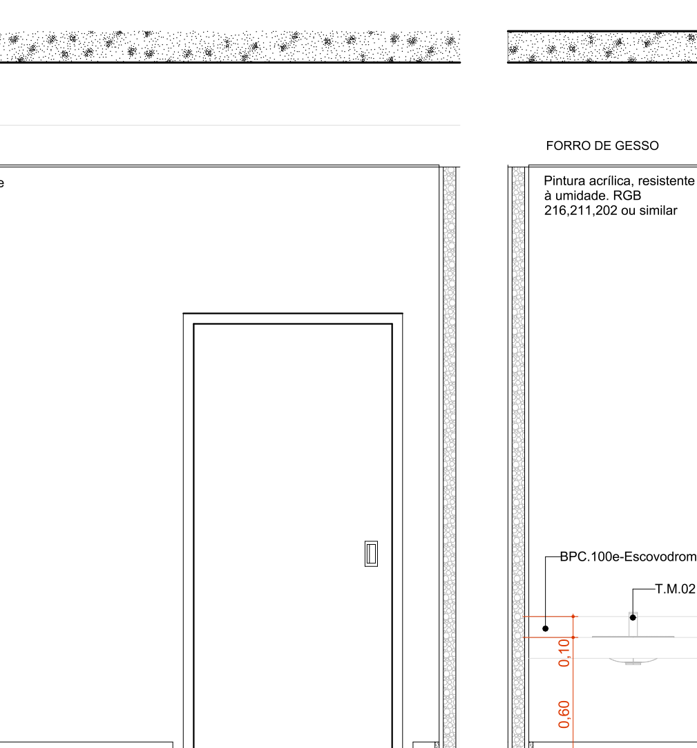
A.M.13 VISTA 3 Escala:1:25
