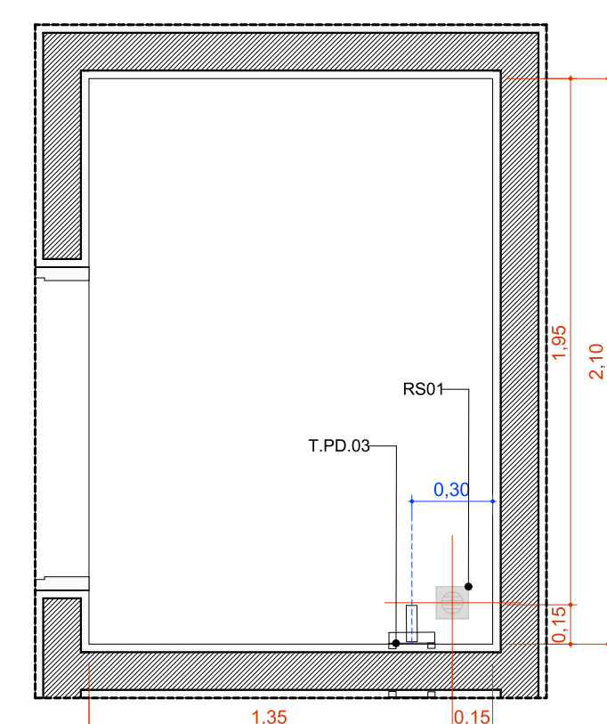
A.M.14 Resíduos Contaminado (Grupos A e E) Escala:1:25
