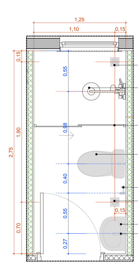
A.M.09 Banh. Func. Fem. Escala:1:25
