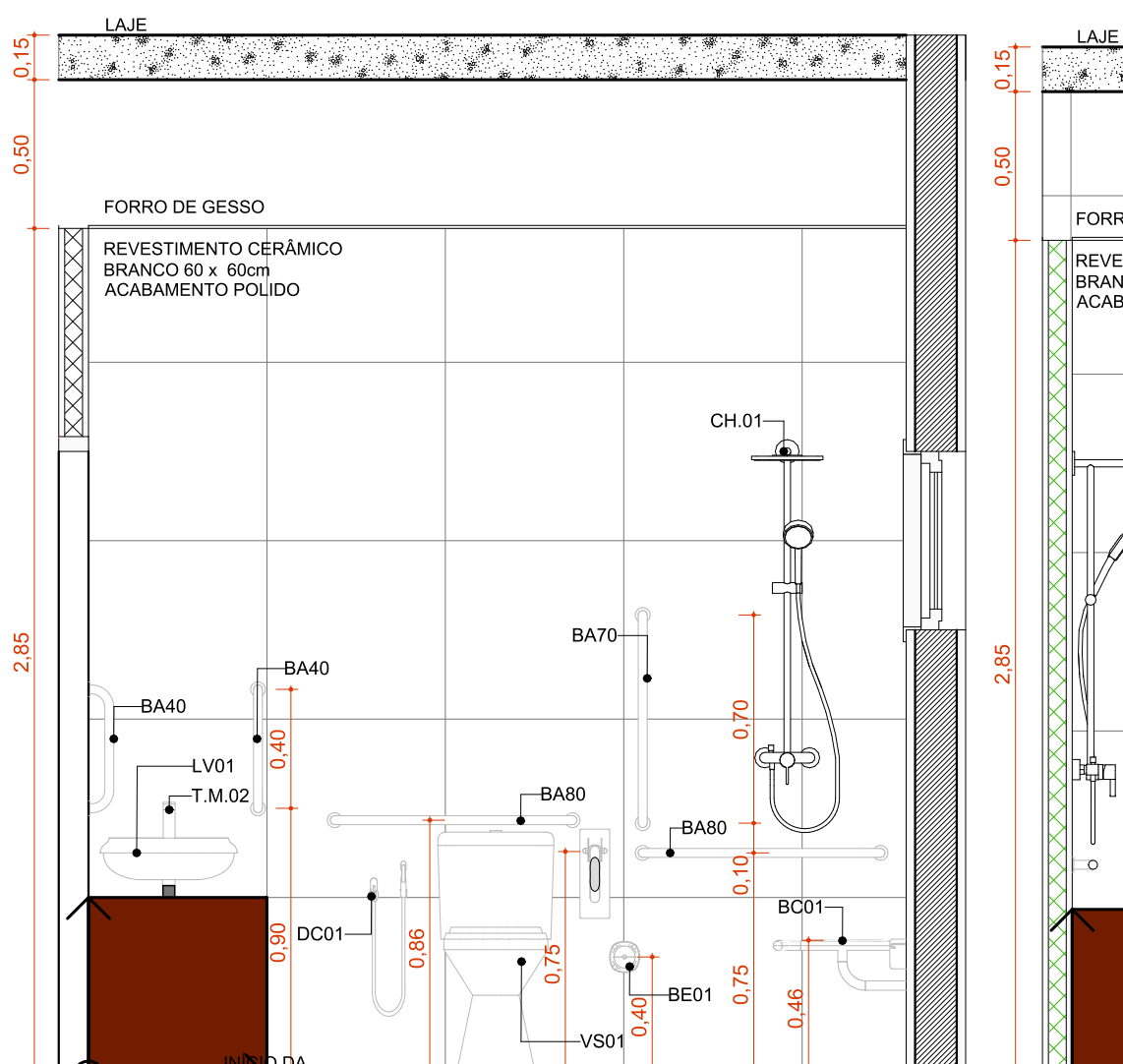
A.M.10 VISTA 1 Escala:1:25
